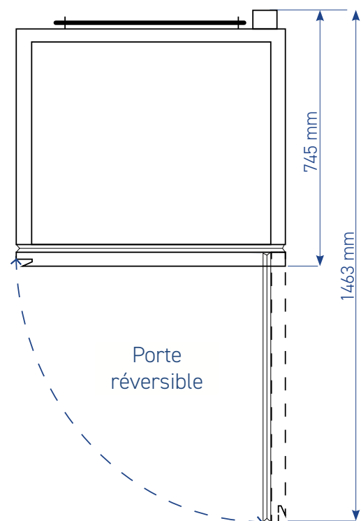
ENCOMBREMENT PORTE OUVERTE
