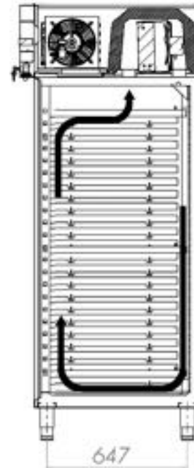
SECTION A-A
