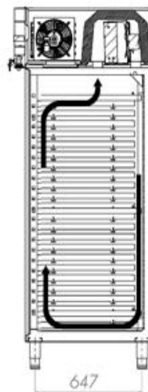
SECTION A-A
